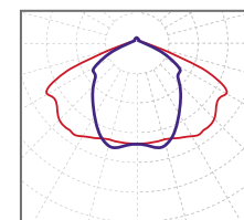
полуширокая осевая КСС 140°x95°
