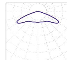
широкая круглосимметричная КСС 140°
