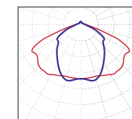
полуширокая осевая КСС 140°x95°
